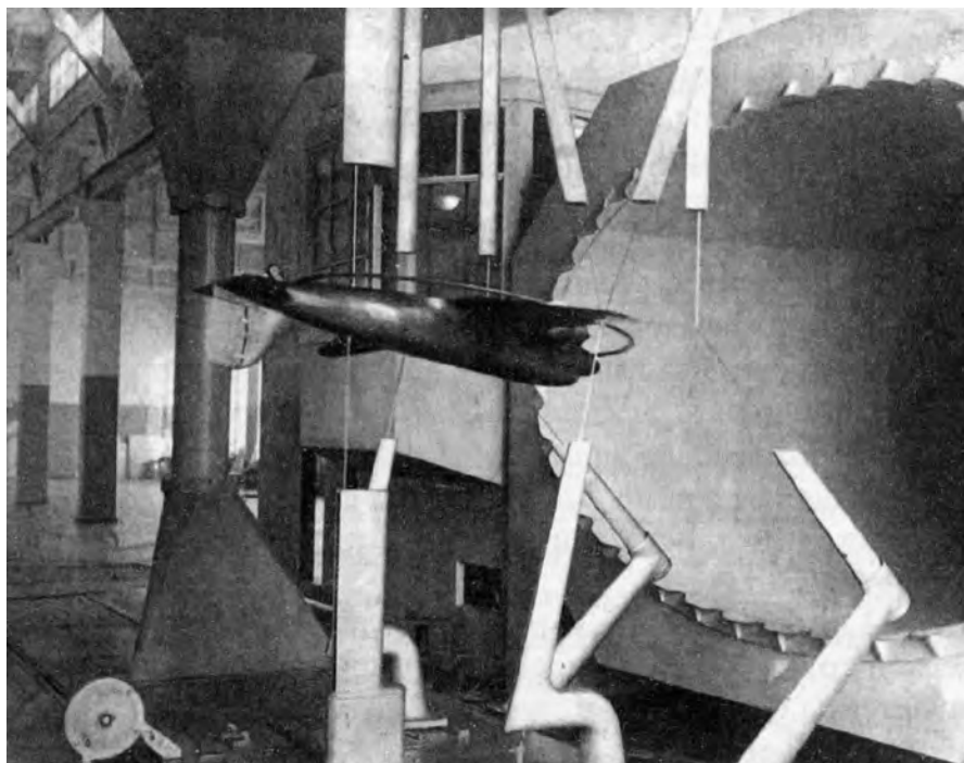
Продувка модели самолёта в аэродинамической трубе Т-203 (Музей Новосибирска)
