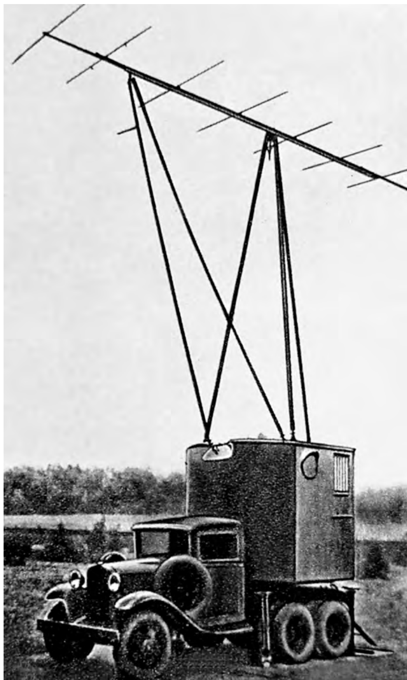
Радиоуправлятель самолётов РУС-2 «Редут» (НИИИП-НЗиК.рф)
