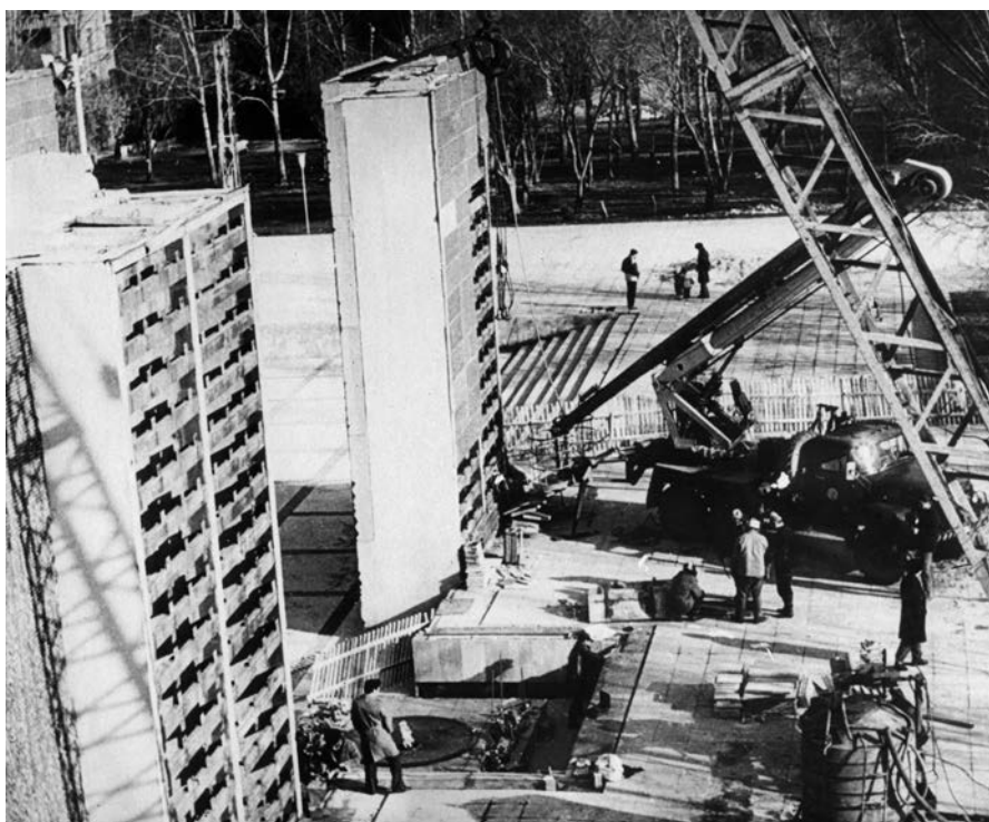
Монтаж пилонов (Музей Новосибирска)
