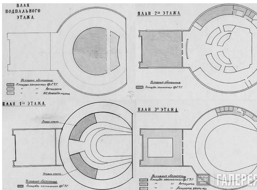
Планы-кальки оперного театра в Новосибирске. 1943 год 14
