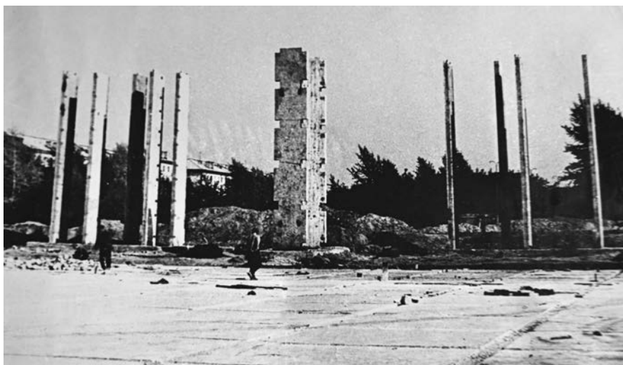
Возведение каркаса пилонов (Музей Новосибирска)
